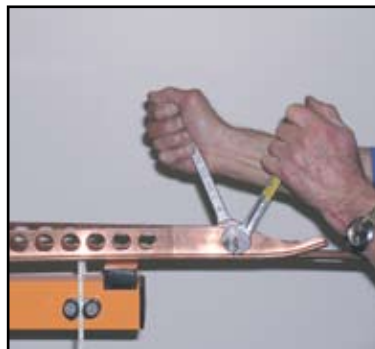
17. Ender og kontramutter trekkes til med 50 Nm.
