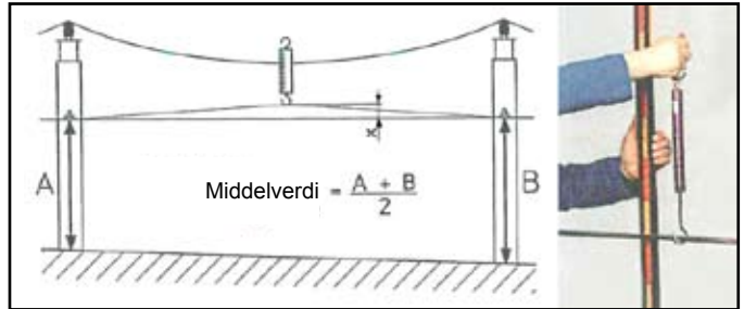
2. Bestem innbyggingshøyde (middelverdi + forhåndløft x). (Bestem x ut fra tabell eller ved hjelp av fjærvekt.)
