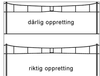
23. De neste 3 hengenetråder på hver side av SI må etterjusteres.
