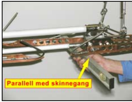
19. Kontrollér innstilling av meier.
