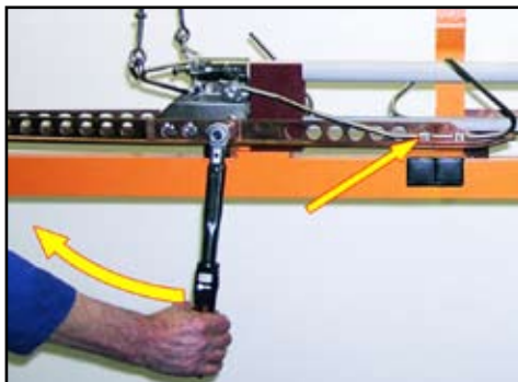
16. Trekk til med 50 Nm.
