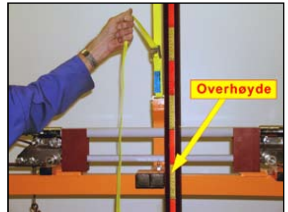
13. Ønsket forhåndløft=overhøyde, stilles inn.
