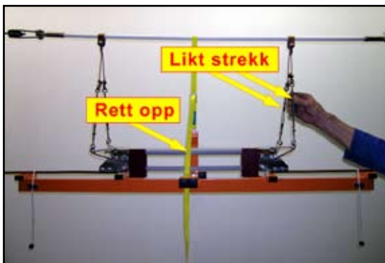
14. Opphengsliner monteres og innjusteres.
