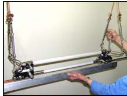
11. Forspenning stilles inn.
