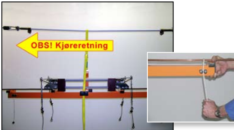
12. Montér hjelpeverktøy. Fiksér line på begge sider.
